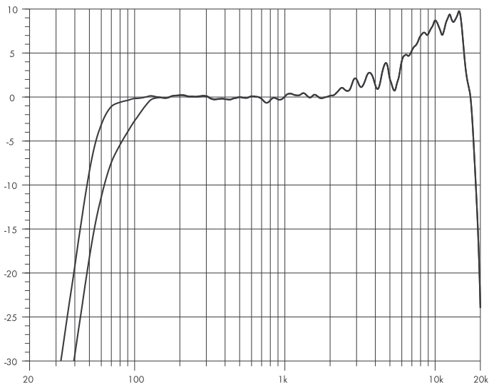
KSL12: Respuesta de frecuencia*, modos Standard y CUT
