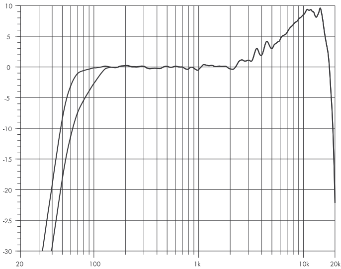
KSL8: Respuesta de frecuencia*, modos Standard y CUT
