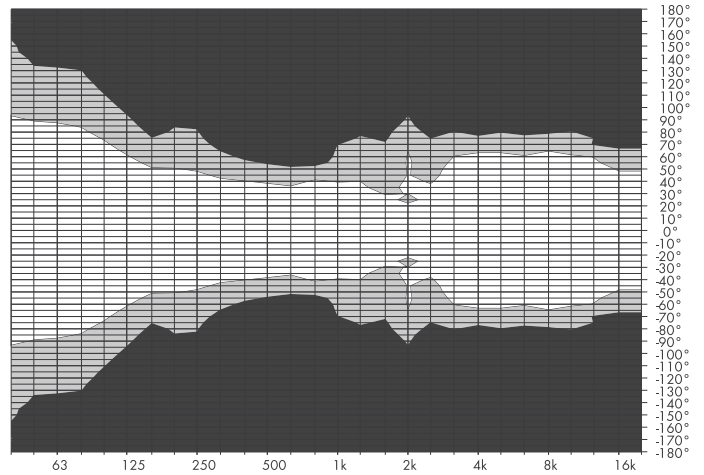
Diagrama de isobara horizontal de KSL12
