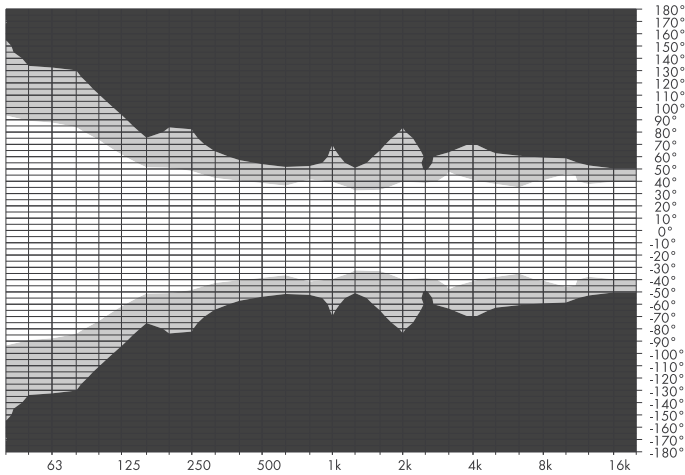
Diagrama de isobara horizontal de KSL8
