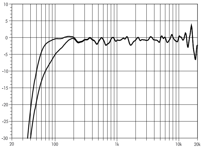
Fig. 17: Respuesta de frecuencia de 10S, ajustes estándar y CUT
