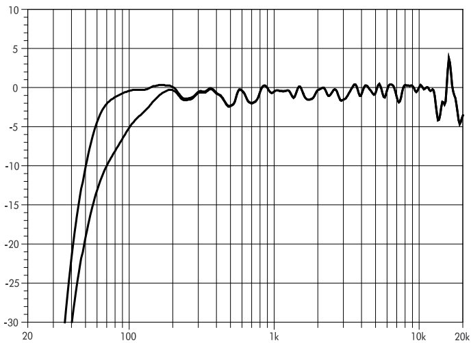
Fig. 18: Respuesta de frecuencia de 10S-D, ajustes estándar y CUT
