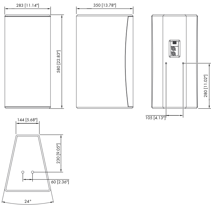
Fig. 19: Dimensiones de la caja de 10S/10S-D en mm [pulgadas]
