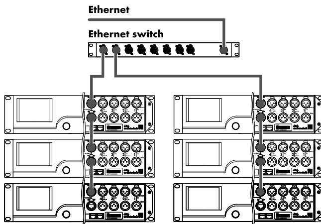
Topología combinada
