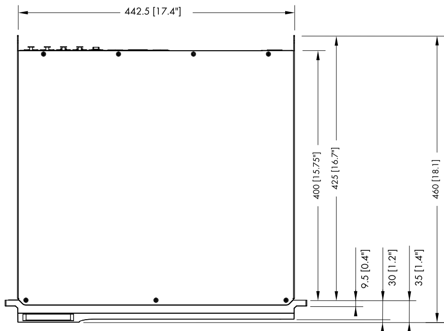
Dimensiones de la caja de D20 en mm [pulg.]
