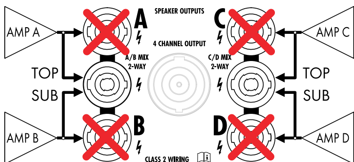
2 x modo Mix TOP/SUB
