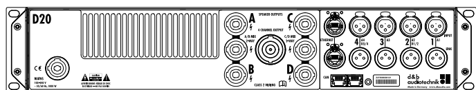
Vista posterior de D20
