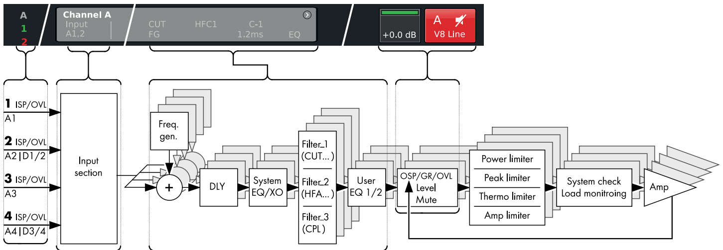
Diagrama esquemático de la hilera de canales D20 (cadena de señal)
