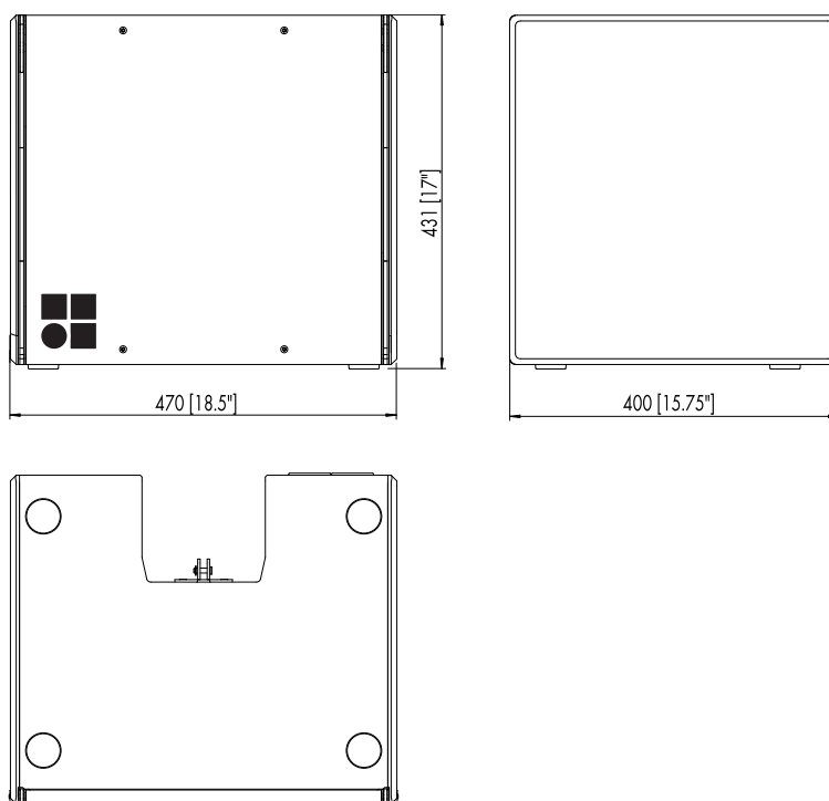
Fig. 5: Dimensiones de la caja de Ti-SUB en mm [pulgadas]
