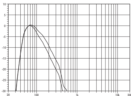
Fig. 4: Respuesta de frecuencia de Ti-SUB, ajustes estándar y 100 Hz
